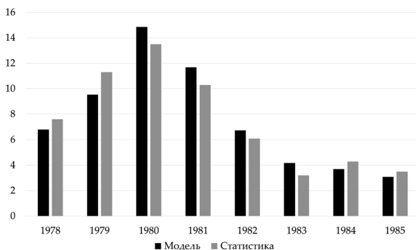
Рис. 9б. Соответствие настроенной модели ПРВ с наблюдаемой инфляцией США (с учетом импорта)
