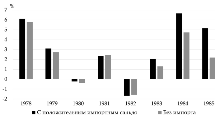
Рис. 9б. Соответствие настроенной модели ПРВ с наблюдаемой инфляцией США (с учетом импорта)
